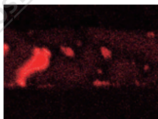
Mg Ka1_2
