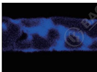
Zn Ka1
