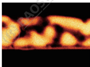
Al Ka1
