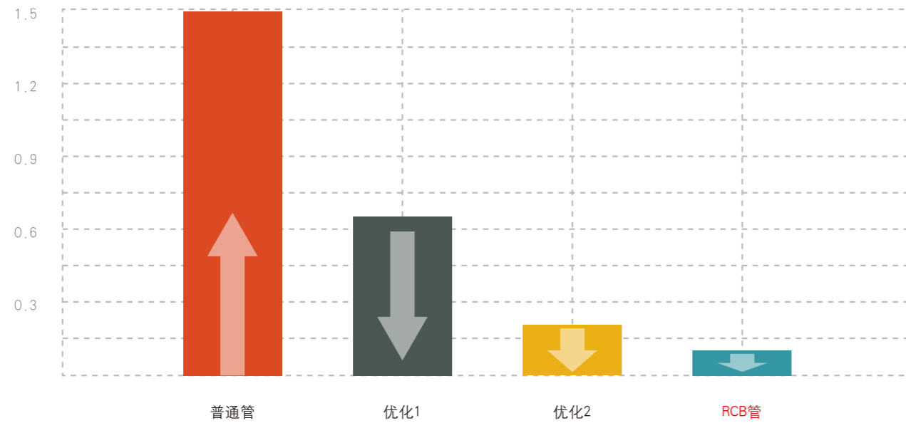
SRB工况局部腐蚀速率 (mm/a)
